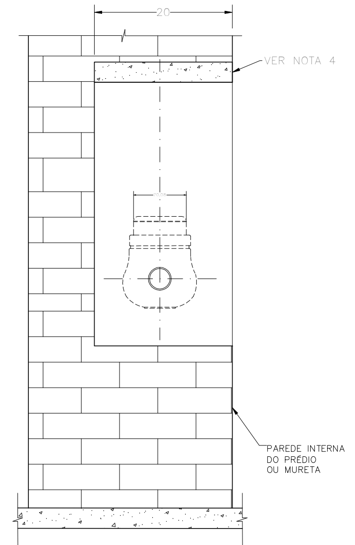
CORTE A-A
