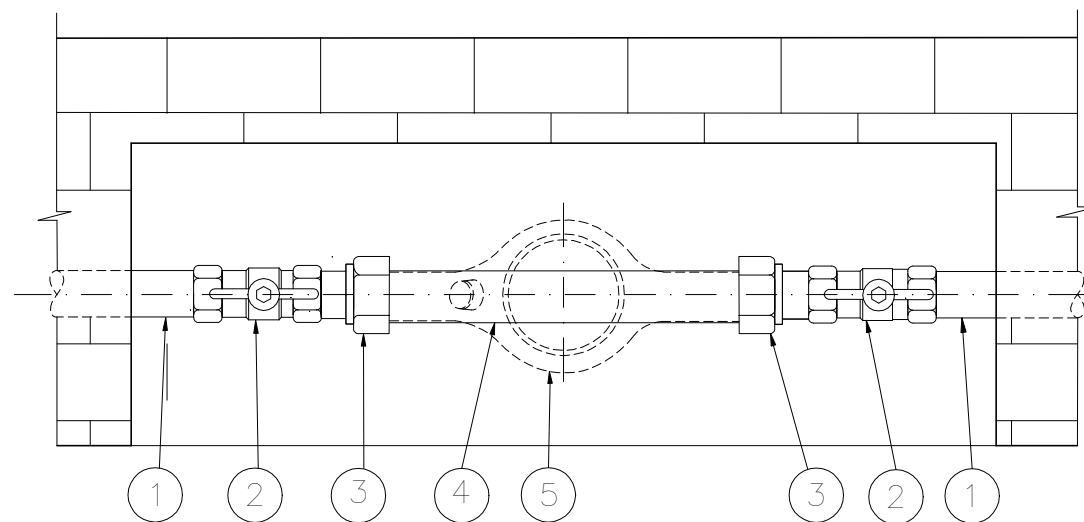
PLANTA
