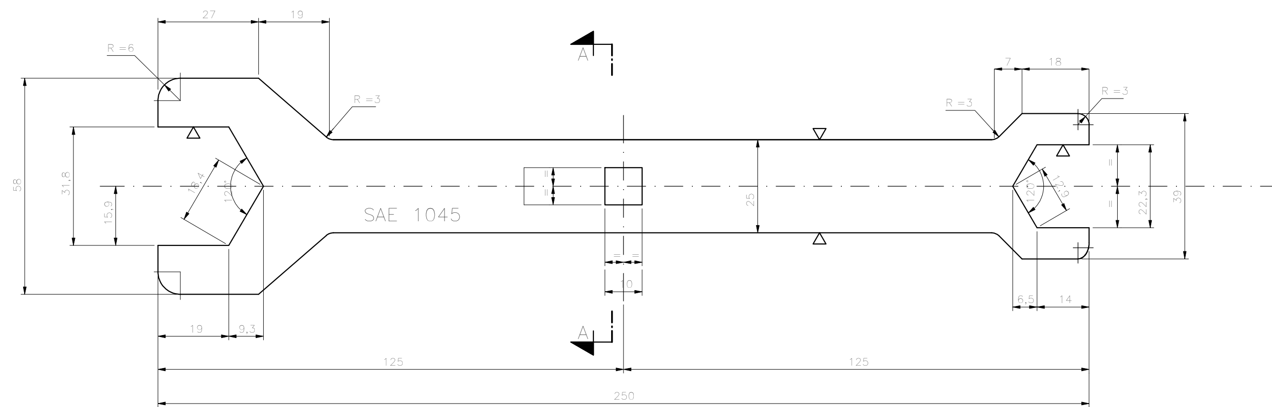
PLANTA ESC. 1:1
